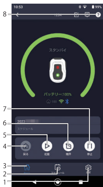
ホーム画面
