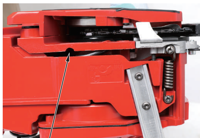
オイル吐出量調整ネジ
